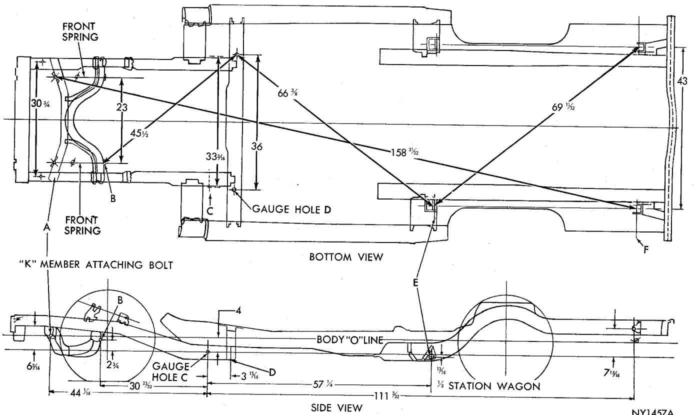
Fig. 199—Body Frame Dimensions (AV Models)
